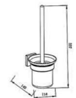
JY12 Toilet Brush Holder 马桶刷
