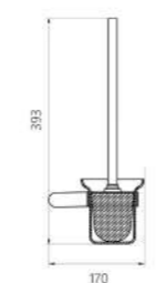
ZFF4 Toilet Brush Holder 马桶刷
